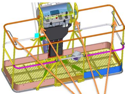
Участки ограждения, обеспечивающие защиту рук от опасности
