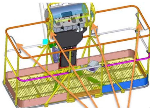
Участки ограждения, защищающие руки от опасности
